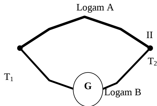
Gb.2 ; Rangkaian termokopel dengan galvanometer
