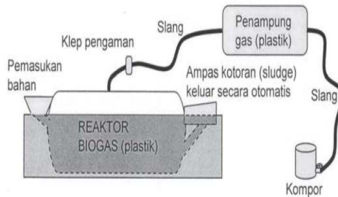
Gambar 2 Instalasi Reaktor Biogas Skala Rumah Tangga
