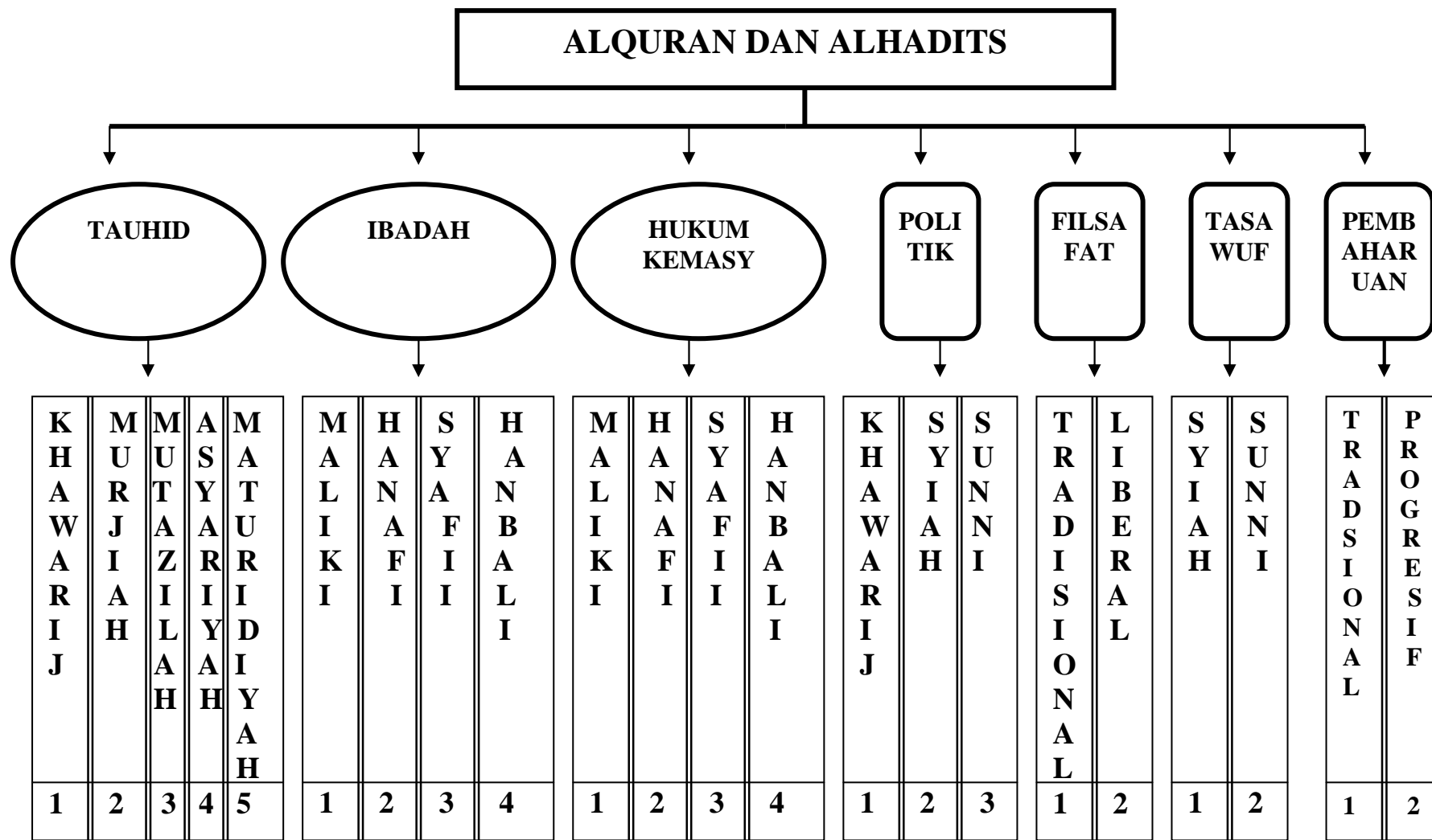
Gambar 4: Skema ilmu keislaman dan aliran-alairan dalam Islam Sumber: Akal dan Wahyu dalam Islam, Nasution, Jakarta: UI.Press 1986
